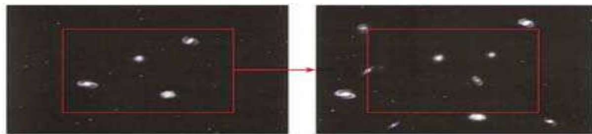
► Figura ilustrează că distanțele dintre galaxii se află într-o continuă creștere, demonstrând, astfel, că întregul Univers se află în expansiune
