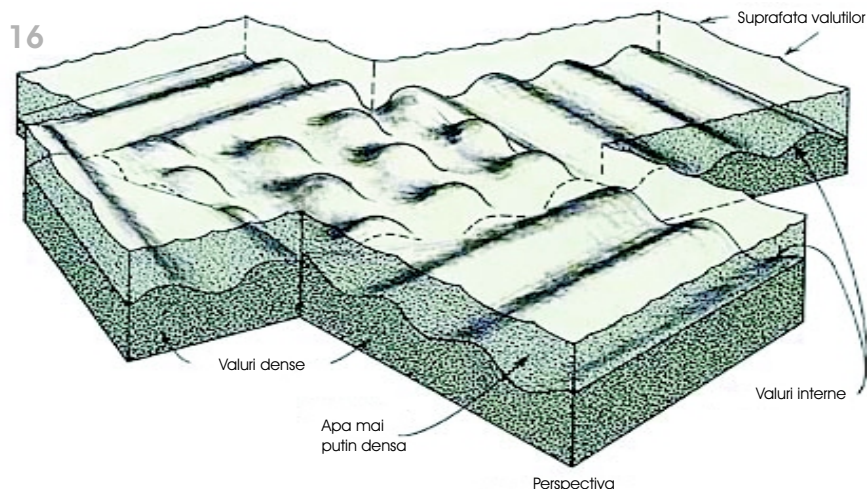
16. Valuri interne formate prin amestecul a doua straturi de apa cu densitati diferite (una este densa, cealalta mai puțin densa, cea de deasupra)
