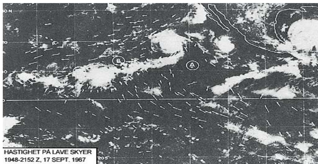
Figur 17: Dette satellittfotoet viser skyer som flyttes mot konvergensområdene (samlingsområdene) B, C og D. Pilene indikerer vindretningen. ( The use of Satellite Pictures in Weather Analysis and Forecasting [Bruken av satellittbilder i væranalyse og værvarsling], Anderson mfl., s. 188)
