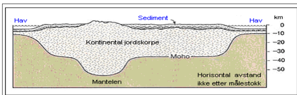
Figur 7: Fjellene har dype røtter under jordens overflate. ( Earth [Jorden], Press og Siever, s. 413)
