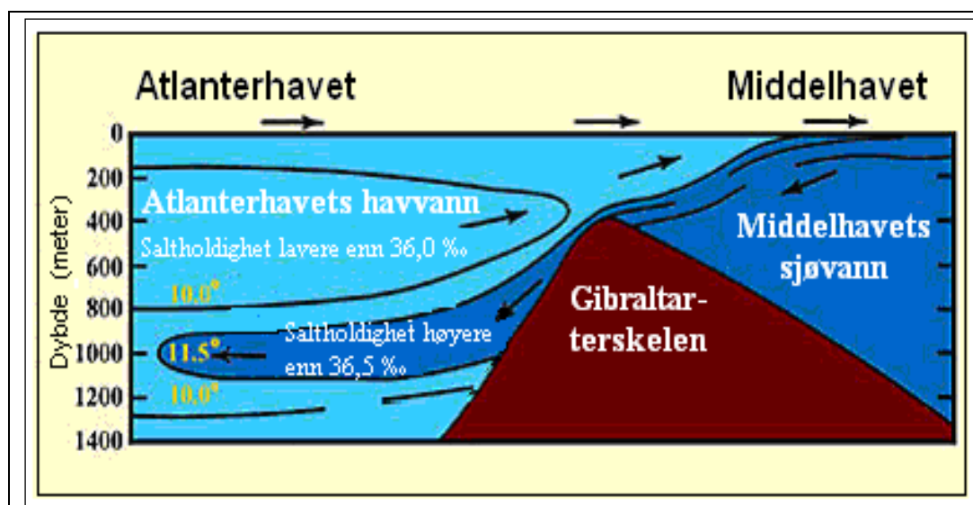
Figur 13: Middelhavets sjøvann entrer Atlanterhavet over Gibraltarterskelen, og beholder sin egen temperatur, saltholdighet og mindre tette karakteregenskap på grunn av barrieren som skiller dem. Temperaturer er oppgitt i grader celsius (°C). ( Marine Geology [Marinegeologi], Kuenen, s. 43, med en liten forbedring)
