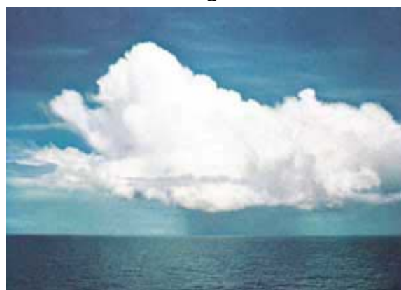
Figur 21: En cumulonimbussky. ( A Colour Guide to Clouds [En fargeguide til skyer], Scorer og Wexler, s. 23)
