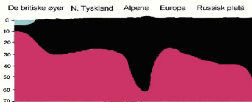
Figur 7: Fjellene har dype røtter under jordens overflate. ( Earth [Jorden], Press og Siever, s. 413)
