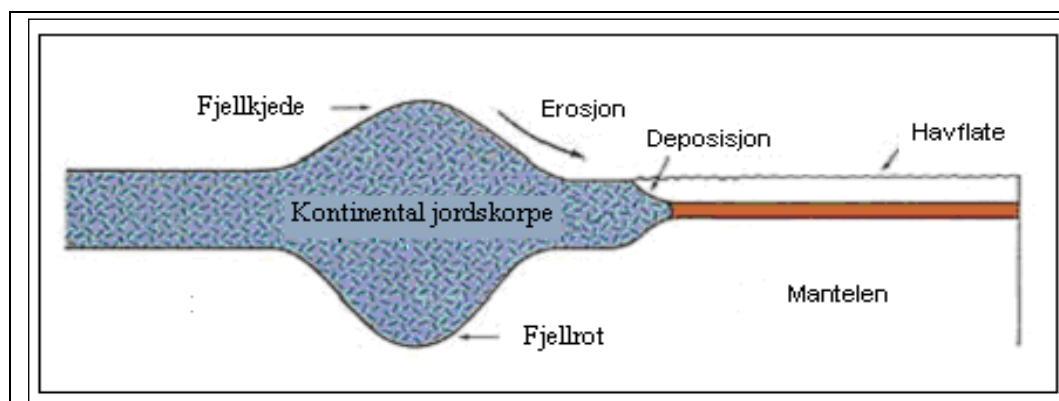
Figur 9: Denne illustrasjonen viser hvordan fjellene på grunn av de dype røttene, har plugglignende form. ( Earth Science [Vitenskapen om jorden], Tarbuck og Lutgens, s. 158)
