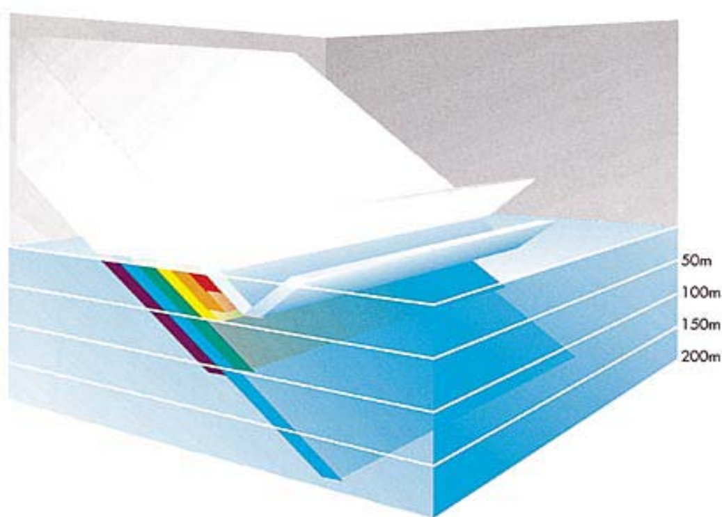
Figur 15: Mellom 3 og 30 prosent av sollyset reflekteres ved havoverflaten. I løpet av de første 200 meterne blir så alle de syv fargene i lysspekteret absorbert en etter en – alle unntatt blått lys. ( Oceans [Hav], Elder og Pernetta, s. 27)
