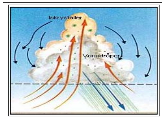
Figur 20: En cumulonimbussky (tordensky). Etter at skyen har blitt stablet opp, kommer det regn ut av den. ( Weather and Climate [Vær og klima], Bodin, s. 123)
