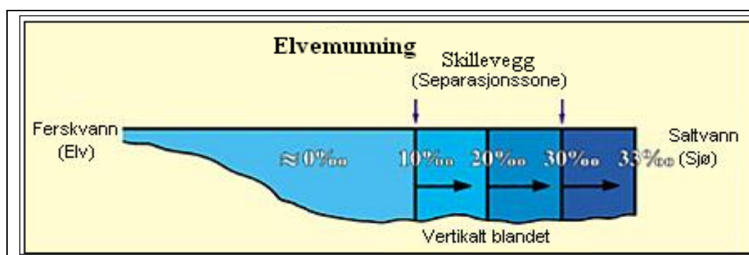
Figur 14: Lengdesnitt som viser saltholdigheten (i promille ‰) i en elvemunning. Her ser vi skilleveggen (separasjonssonen) mellom ferskvann og saltvann. ( Introductory Oceanography [Innledende oseanografi], Thurman, s. 301, med en liten forbedring)
