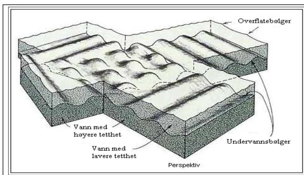
Figur 16: Undervannsbølger på grenseflaten mellom to lag av vann med forskjellig tetthet. Det nedre laget har høyere tetthet, og det øvre laget har lavere tetthet. ( Oceanography [Oseanografi], Gross, s. 204)
