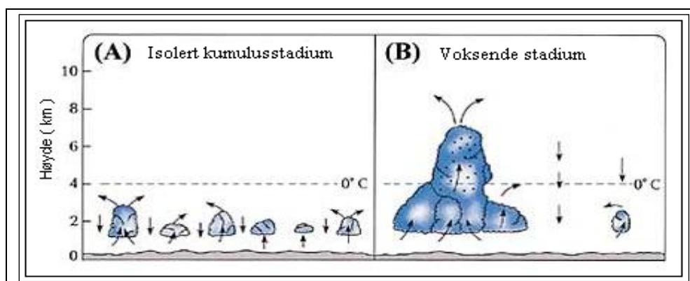
Figur 19: (A) Isolerte smådelar av skyer (cumulusskyer). (B) Når de små skyene samles, øker oppdriften i den større skyen, slik at skyene blir stablet opp. Vanndråper er indikert med •. ( The Atmosphere [Atmosfæren], Anthes mfl., s. 269)
