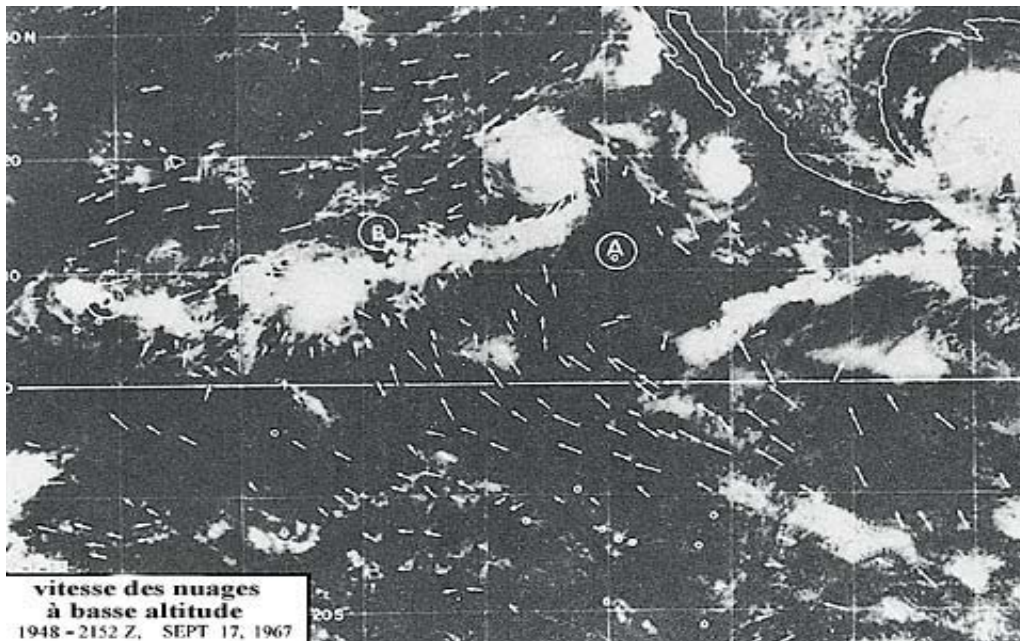
Illustration 17: Photo satellite montrant les nuages se déplaçant vers les aires de convergence B, C, et D. Les flèches indiquent les directions du vent. ( The Use of Satellite Pictures in Weather Analysis and Forecasting [L'utilisation des images satellites dans l'analyse et les prévisions météorologiques], Anderson et al., p. 188.)
